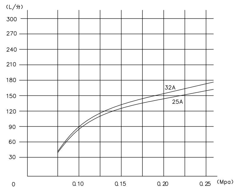
ステンレス吐水口 流量線図
