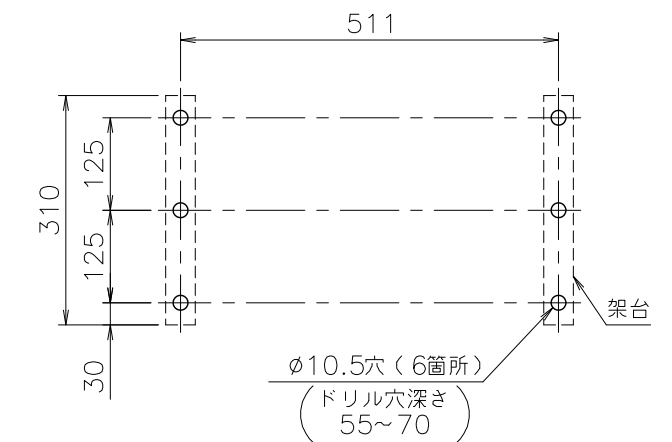
■オールアンカの穴寸法 (尺度 1/10)
