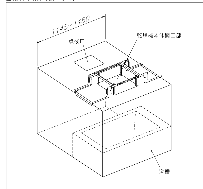
■後付け架台設置参考図
