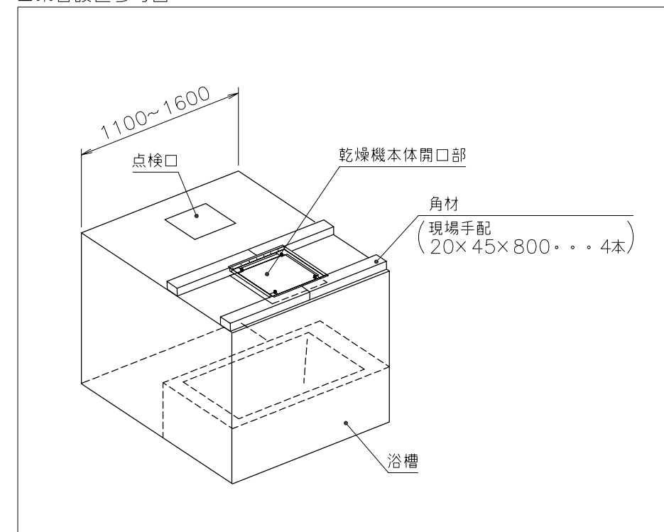
■ 架台設置参考図
