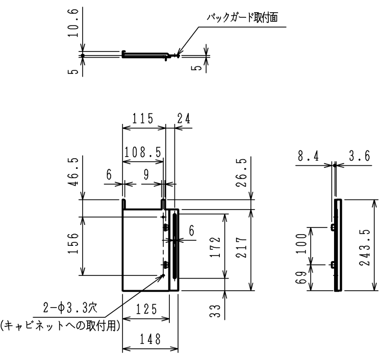
バックガード取付板
