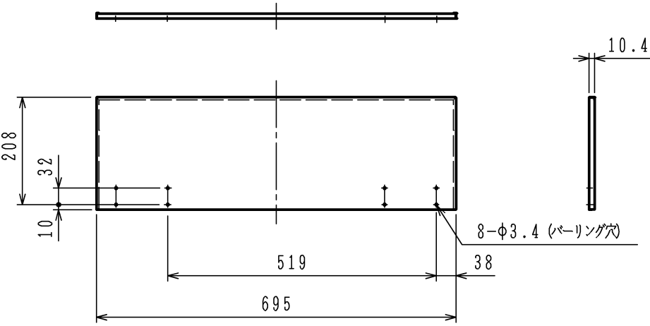
バックガード
