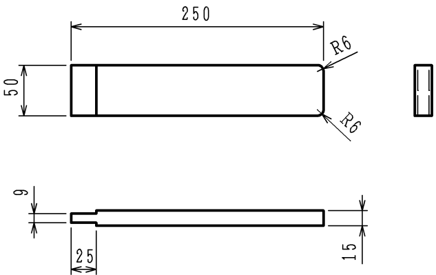
スペーサー
