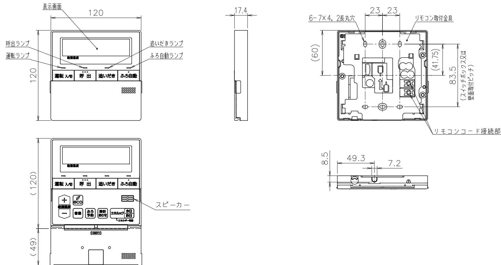
台所リモコン RC-J112ME
