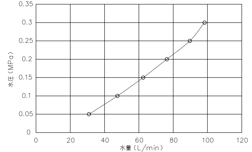
JN-1S-AZ の性能データ (合成 (水 + エア) 流量データ) ※ 水面下 150mm の流量データです。 ※ 二連型 JNW-2S-AZ は下表の流量データ X2 倍です。 ※ 三連型 JNT-2S-AZ は下表の流量データ X3 倍です。
