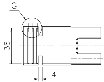
断面E-E
