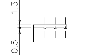
D部詳細図（S= 1／1）
