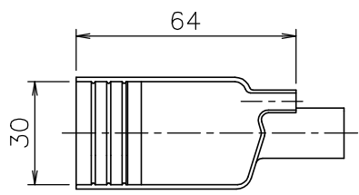
断面C-C
