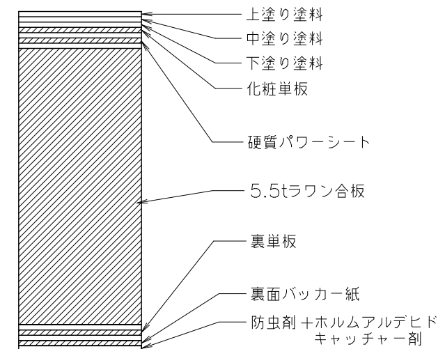
■構成図（6TフローリングH－＊＊）
