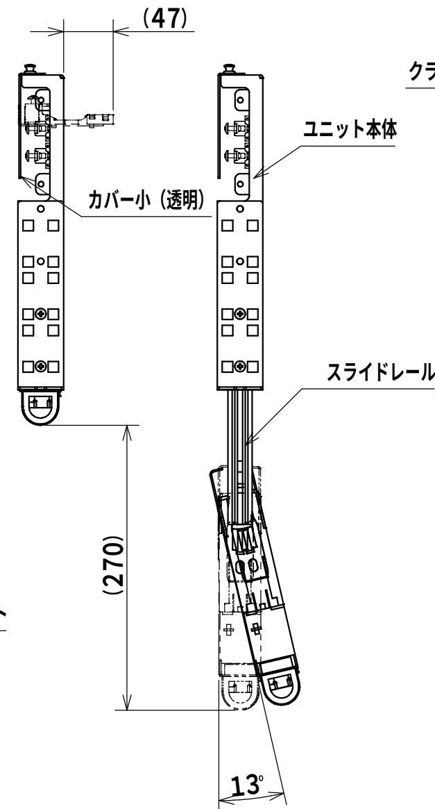
引出しユニット傾斜図
