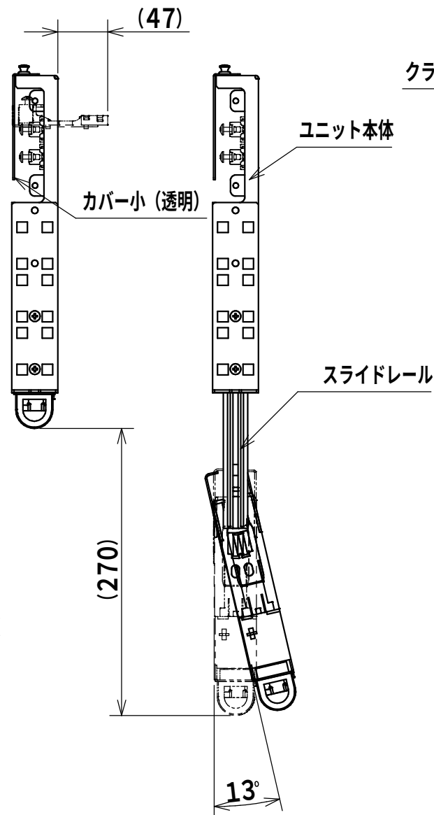
引出しユニット傾斜図
