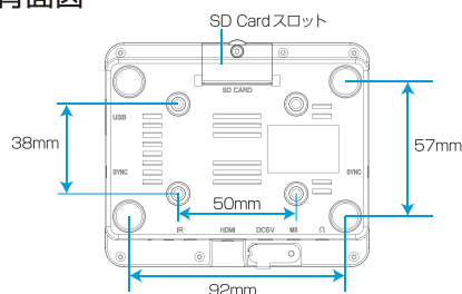
背面図
