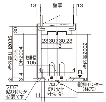
縦断面図
