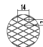
ワジョン ラス網 7×14 (呼称・5メッシュ)
