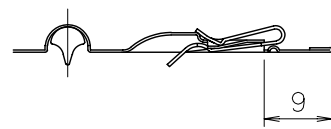
A-A'断面 (S=1:1)
