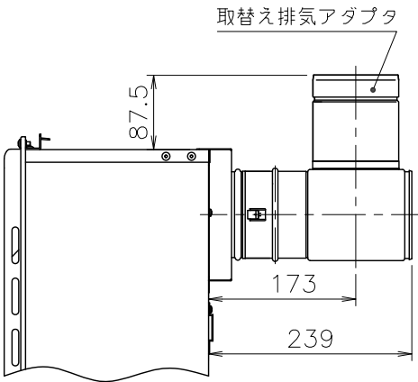
■ 取り付け参考図
