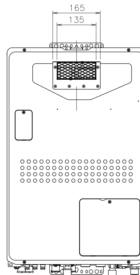
■取付参考図（尺度：1／8）
