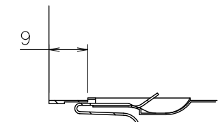
抜止金具拡大図 (S=3:1)
