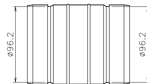
断面図 C-C
