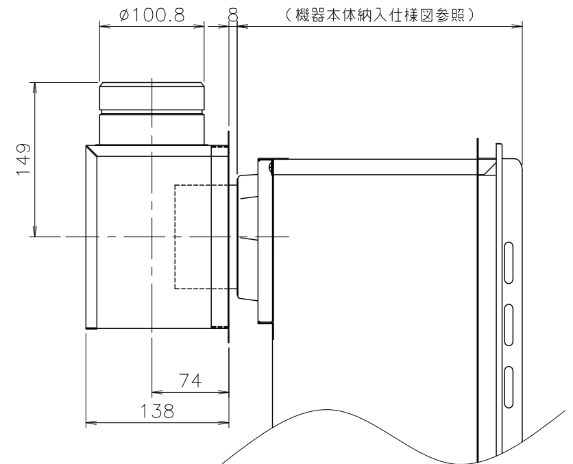
■取付参考図
