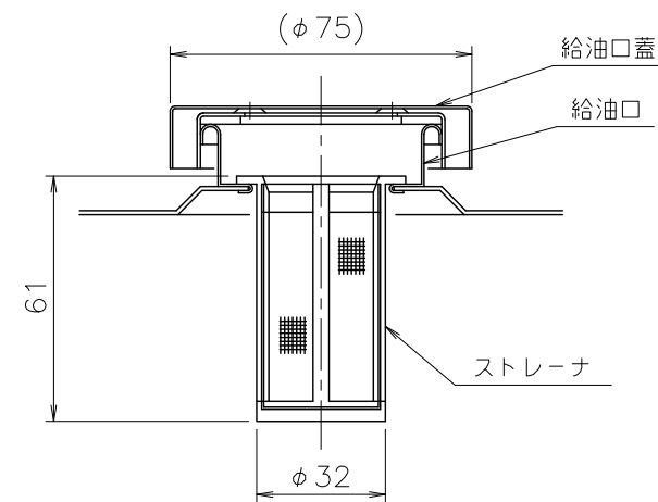
給油口詳細 (S=1/2)
