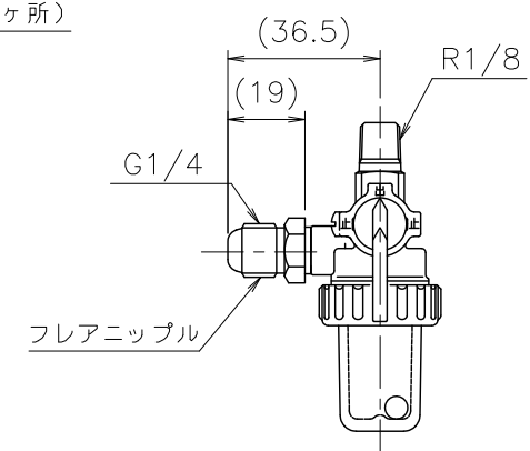
送油バルブ詳細 (S=1/2)
