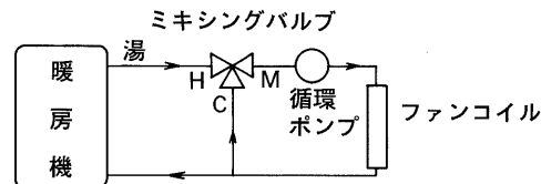
〈配管使用例〉
