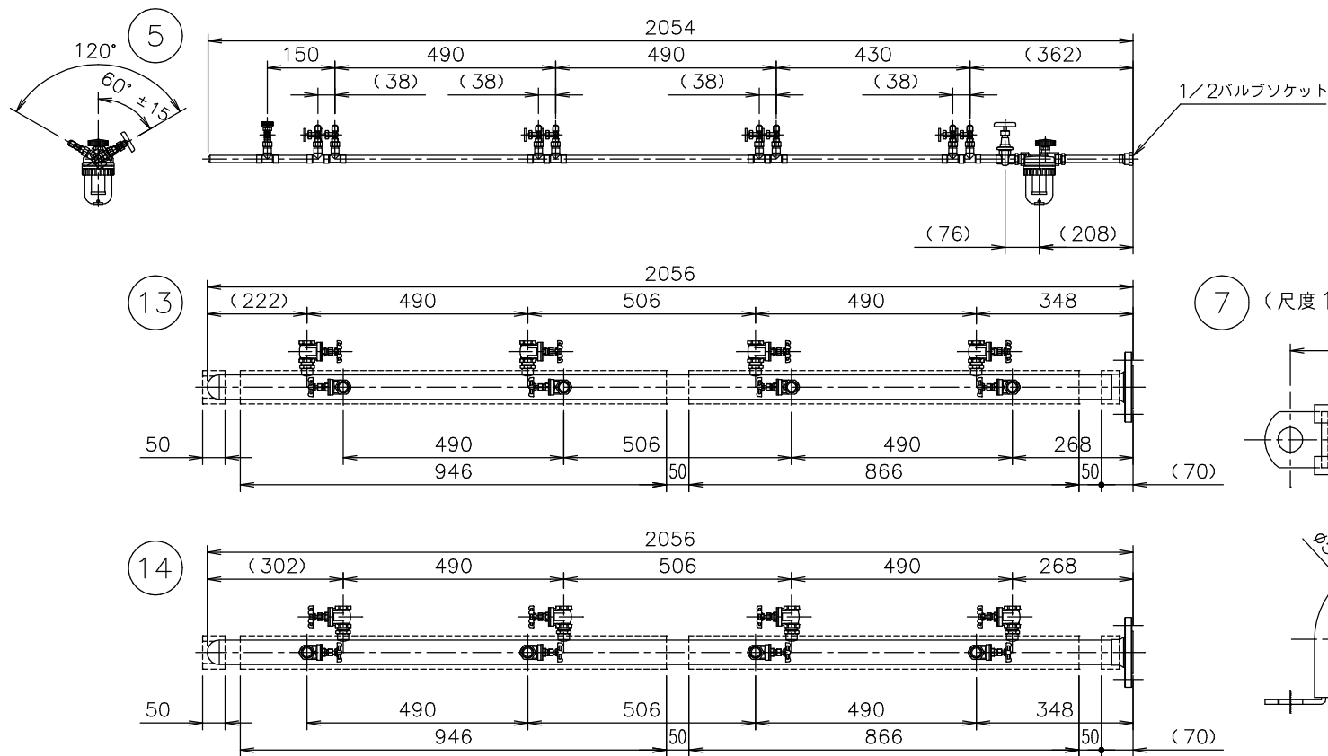
組立参考図
