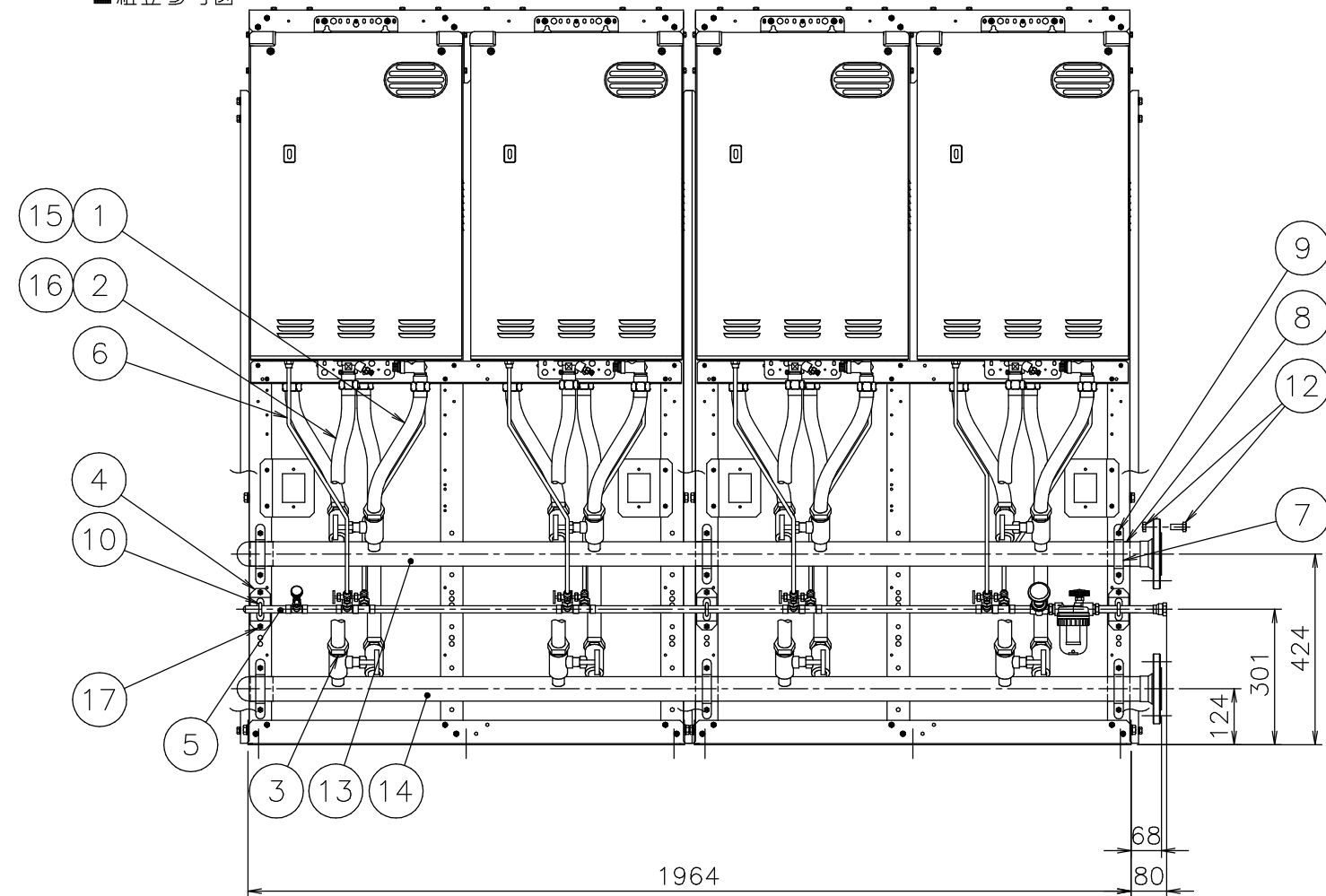
組立参考図
