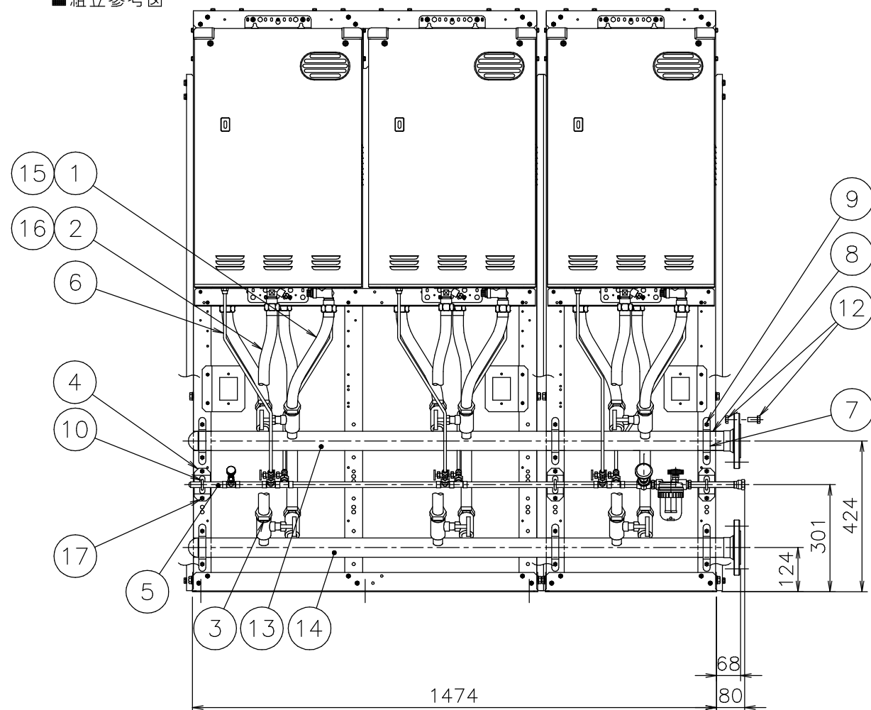
組立参考図
