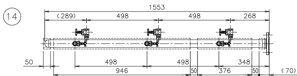
組立参考図
