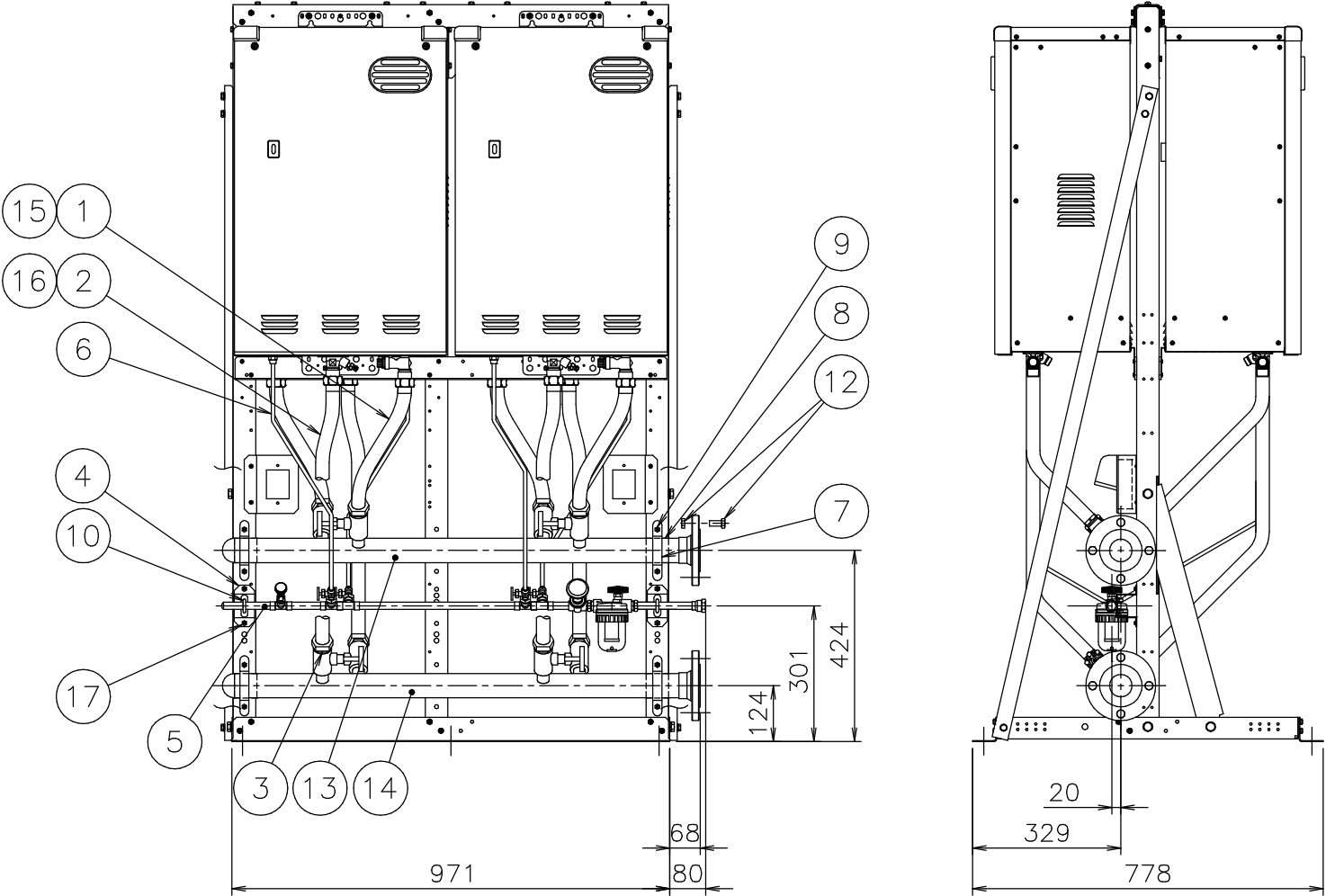
組立参考図
