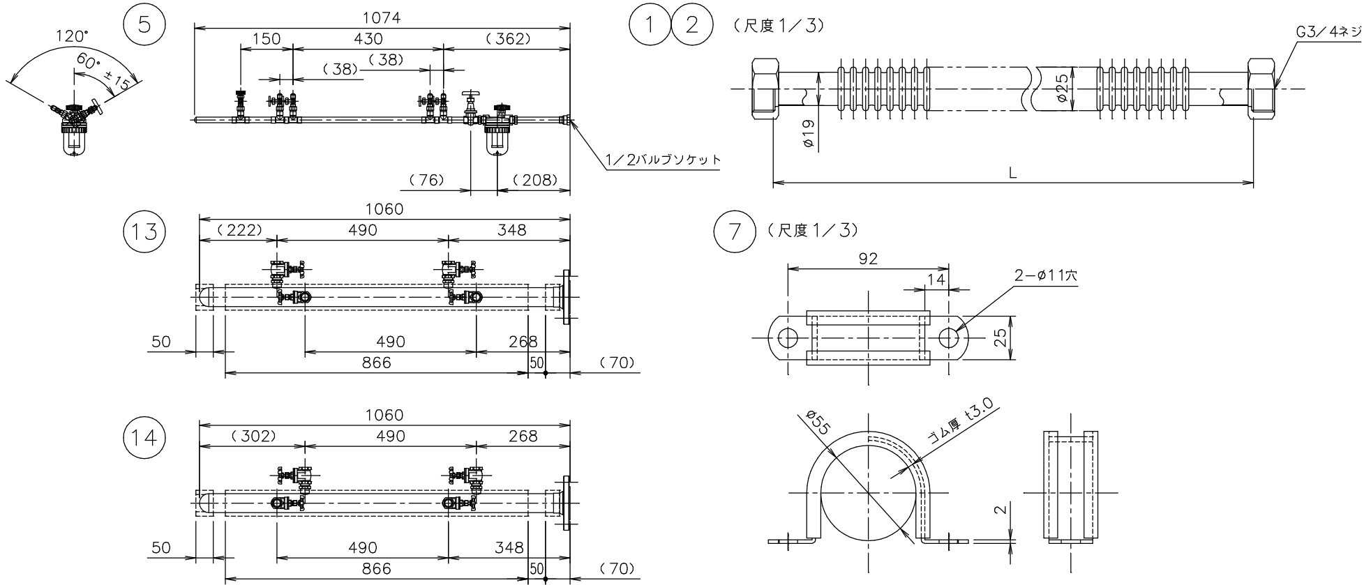
組立参考図
