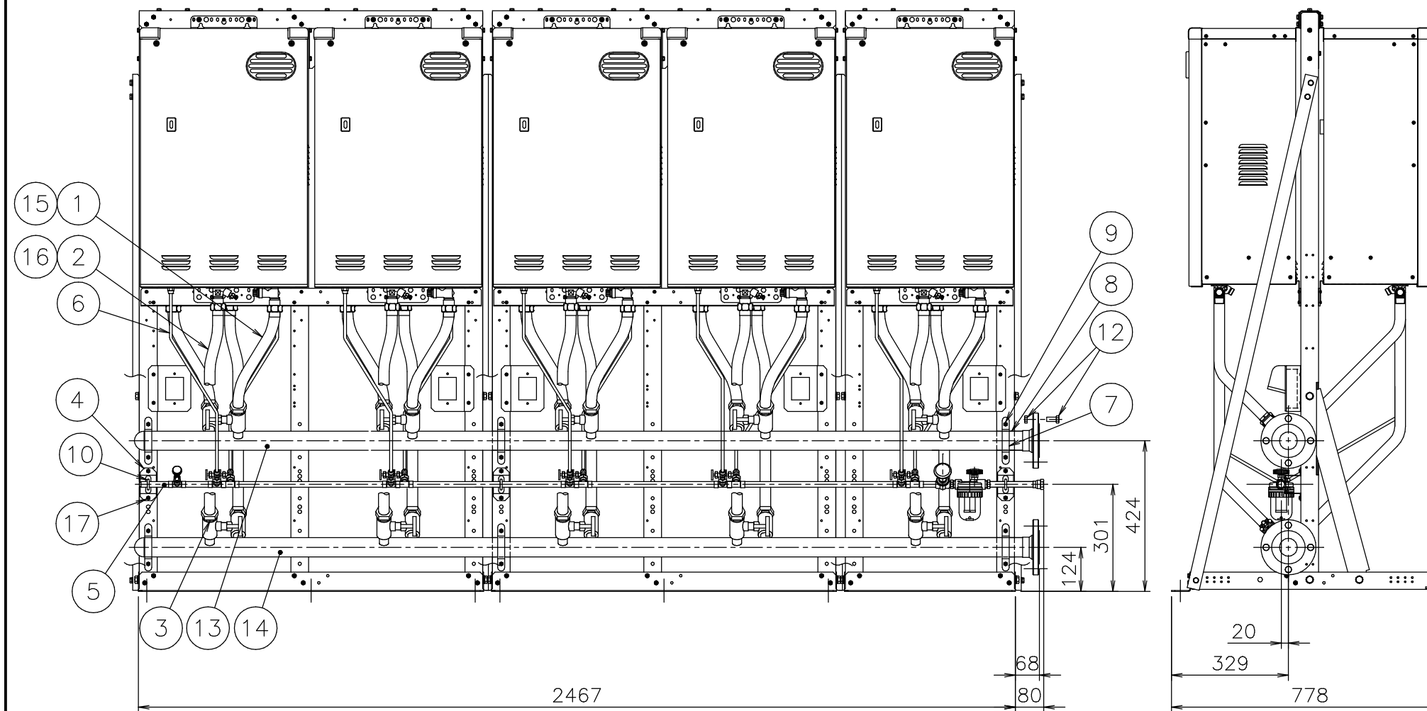
組立参考図
