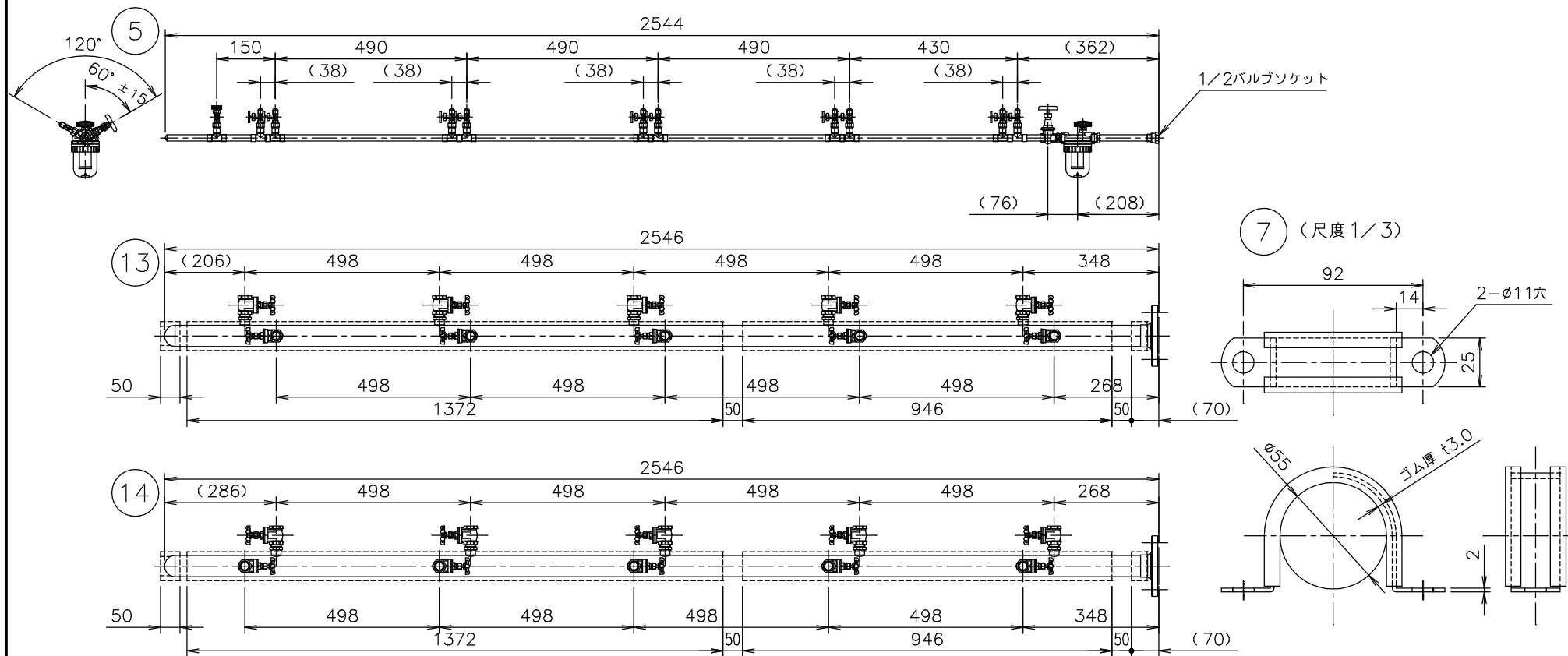
組立参考図
