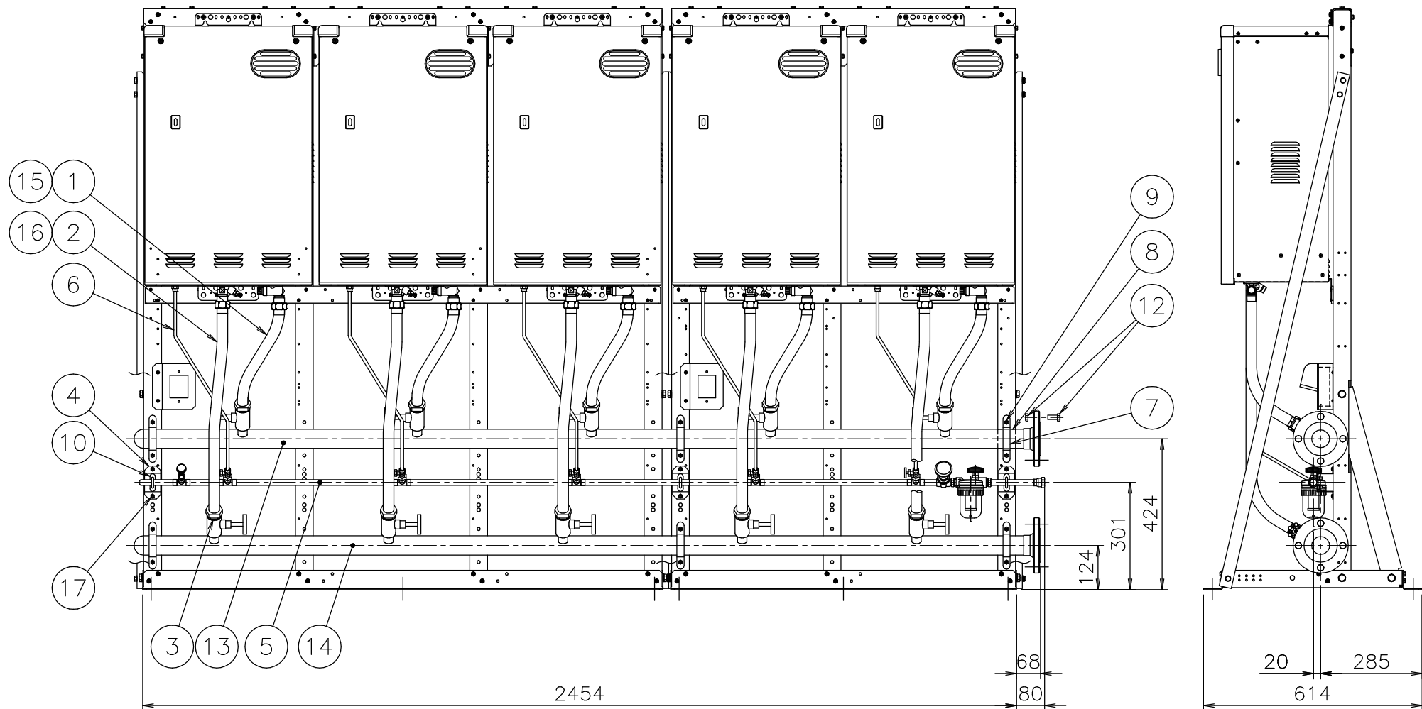
■組立参考図
