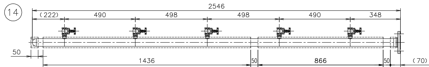
■組立参考図
