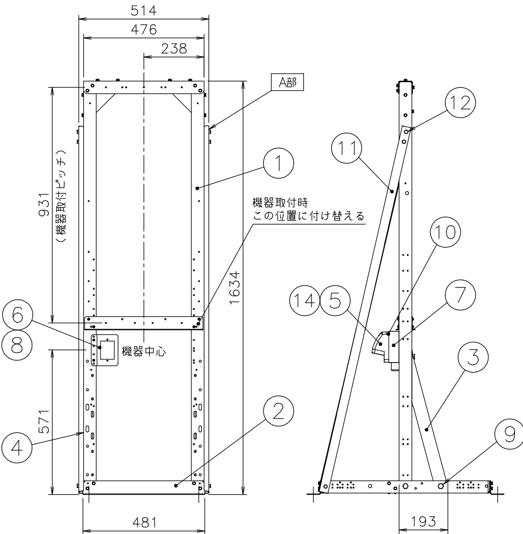
■A部詳細図（尺度1／2）
