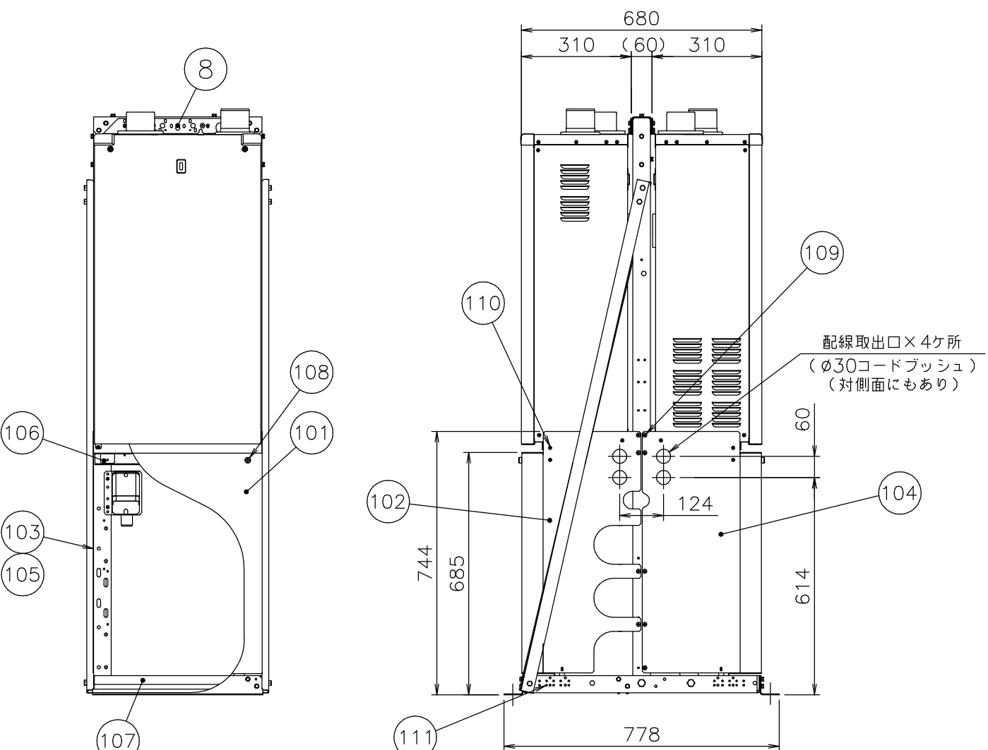
■マルチ架台カバー組立図（※現場組み立てになります）
