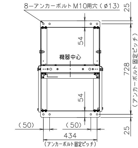
■マルチ架台組立図（※現場組み立てになります）
