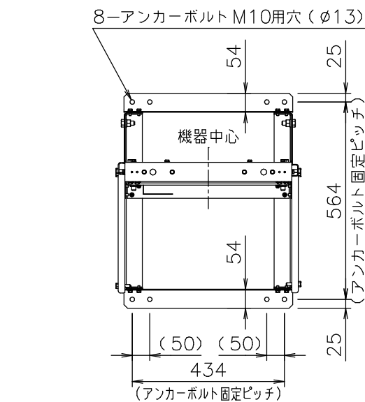
■ マルチ架台組立図（※現場組み立てになります）
