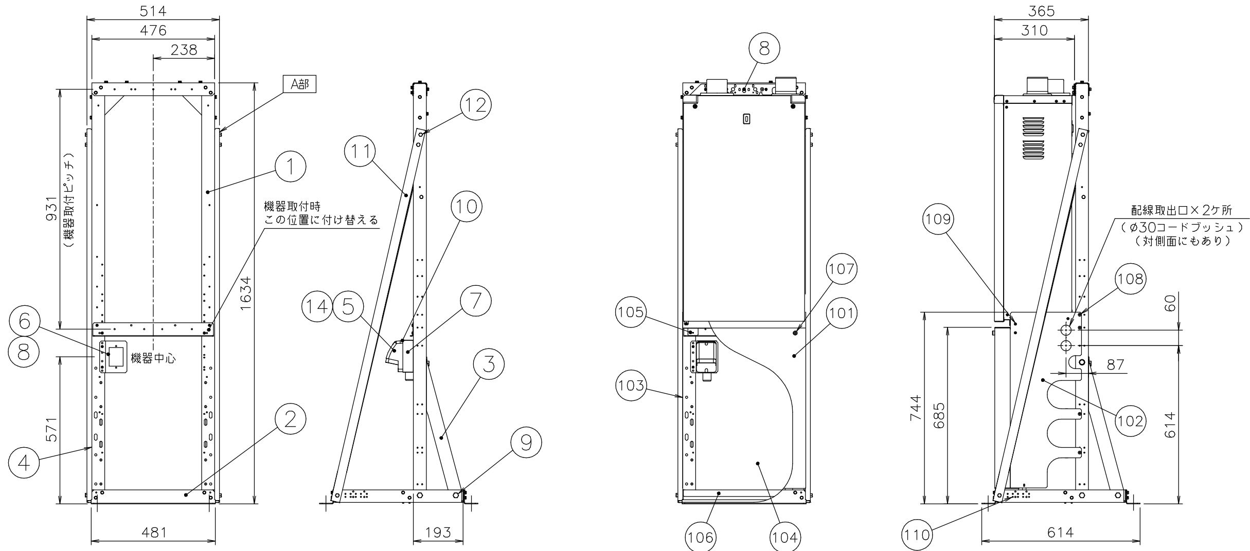
■ マルチ架台カバー組立図（※現場組み立てになります）
