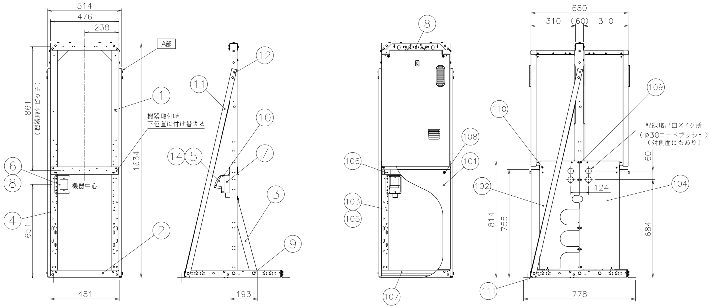
■ マルチ架台カバー組立図（※現場組み立てになります）
