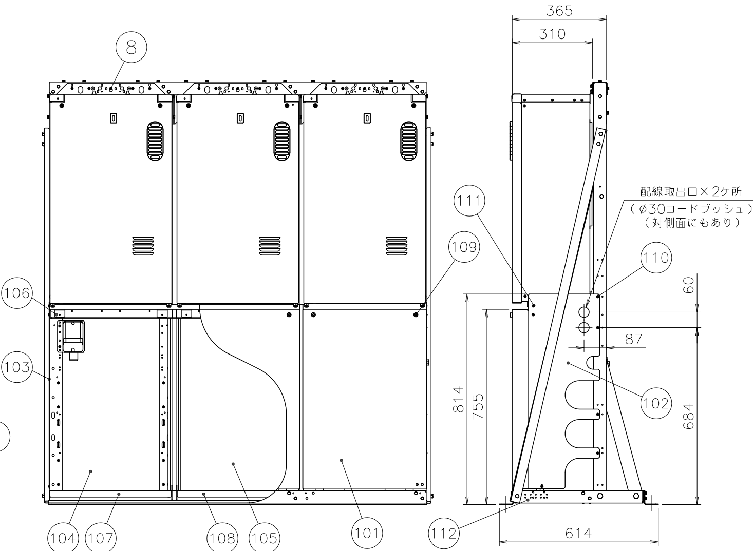
■マルチ架台カバー組立図（※現場組み立てになります）
