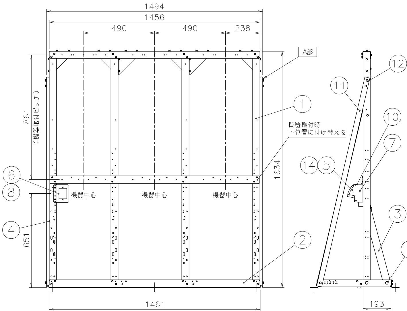
■A部詳細図（尺度1/2）
