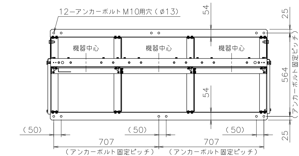
■マルチ架台組立図（※現場組み立てになります）
