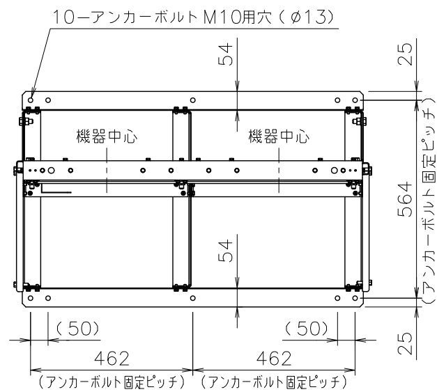
■ マルチ架台組立図（※現場組み立てになります）
