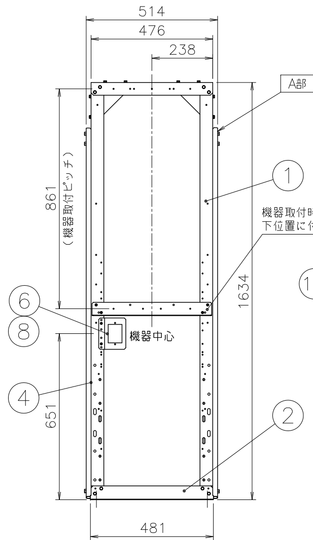
■ A部詳細図（尺度 1／2）
