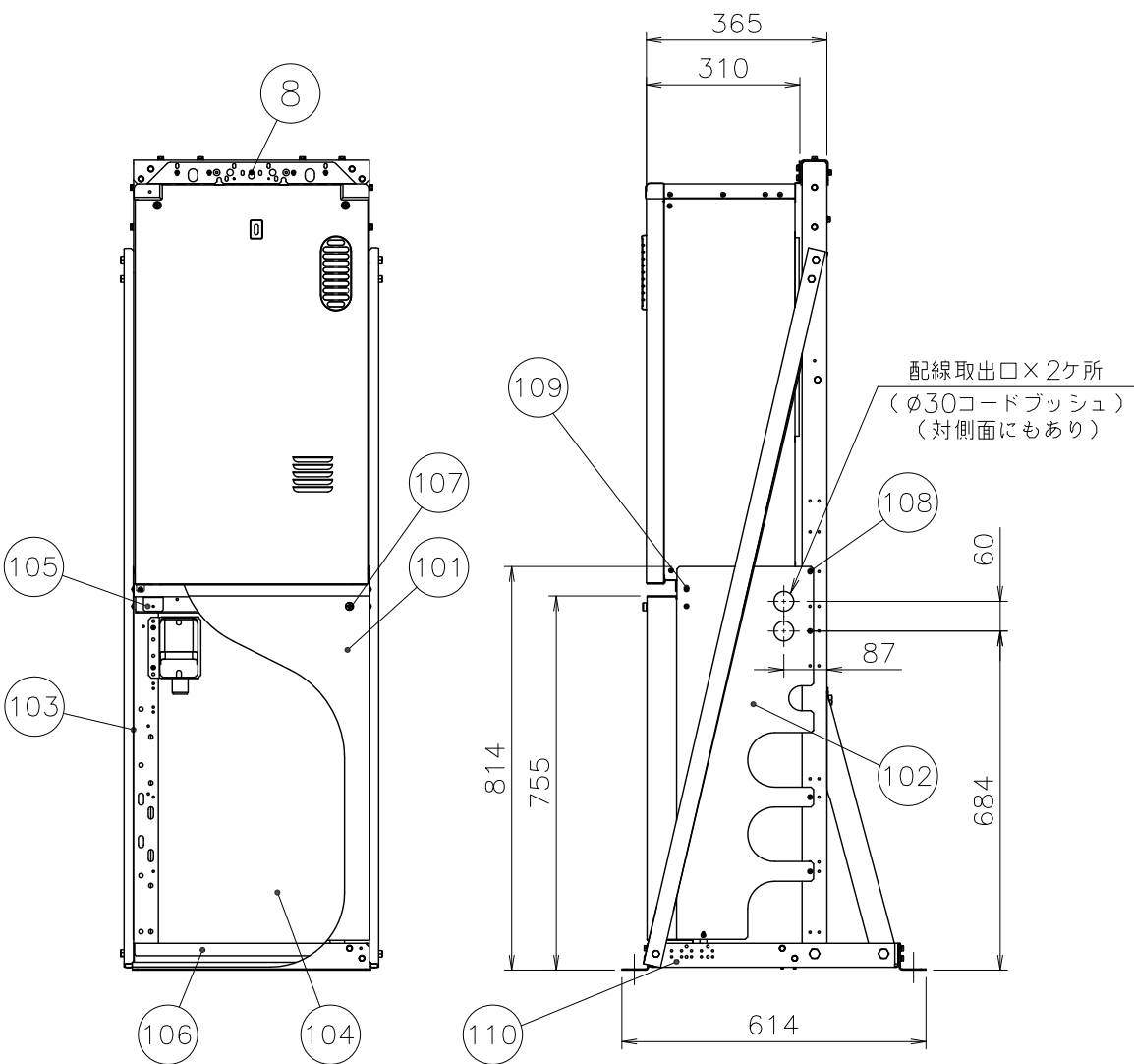
■ マルチ架台カバー組立図（※現場組み立てになります）
