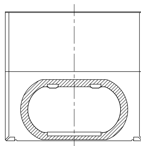
排気カバー裏面 Aから見る (尺度1/3)
