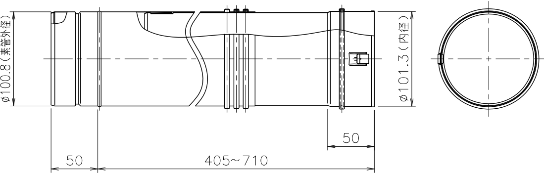
■φ100スライド管 (L405~710) × 1 材質：SUS304 t0.3
