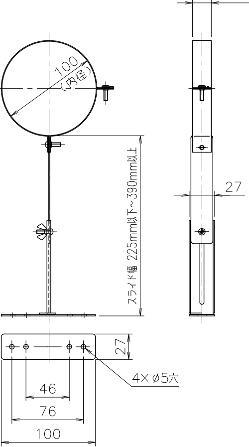
■φ100固定金具 (225~390) × 1 材質：SUS304 t0.8,1.5
