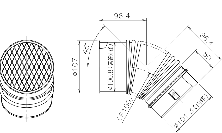
■φ100エルボトップ 45°× 1 材質：SUS304 t0.3
