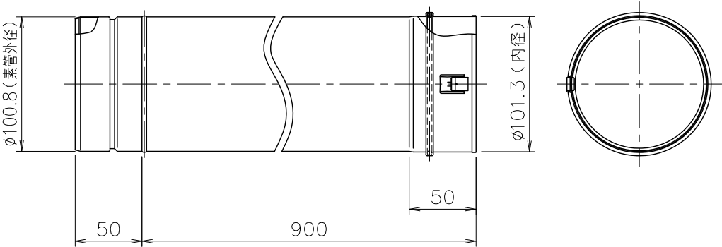
■φ100直管 L900× 1 材質：SUS304 t0.3
