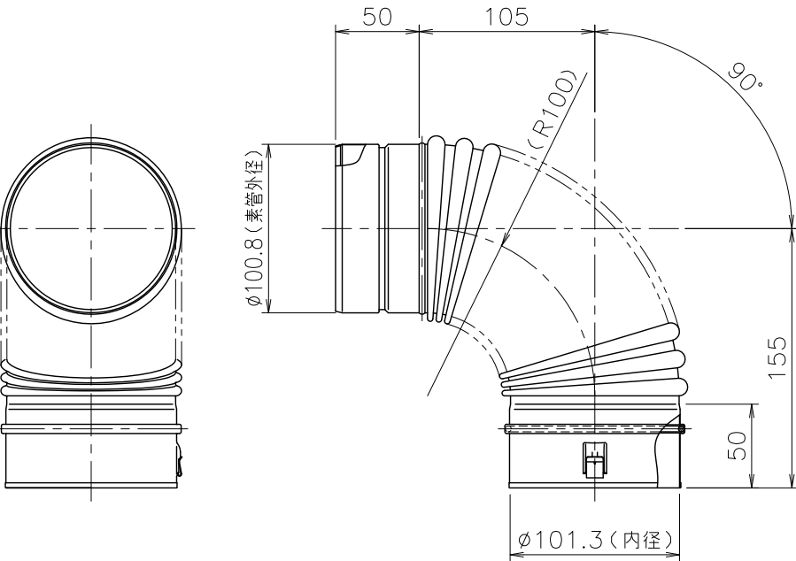
■φ100エルボ 90°× 1 材質：SUS304 t0.3
