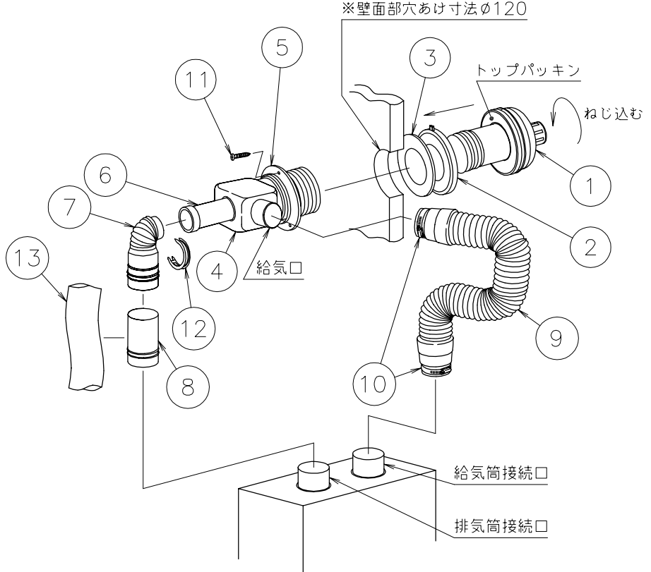
■組立図
