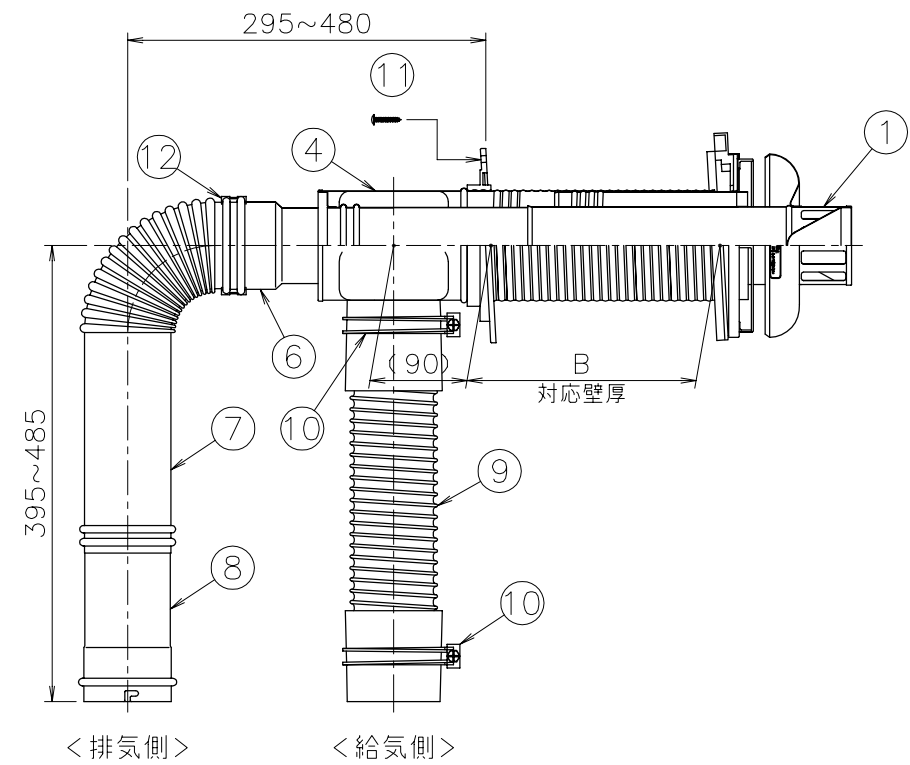
側面図
