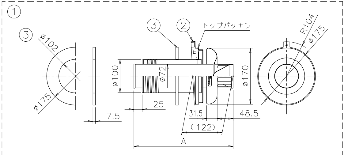
側面図
