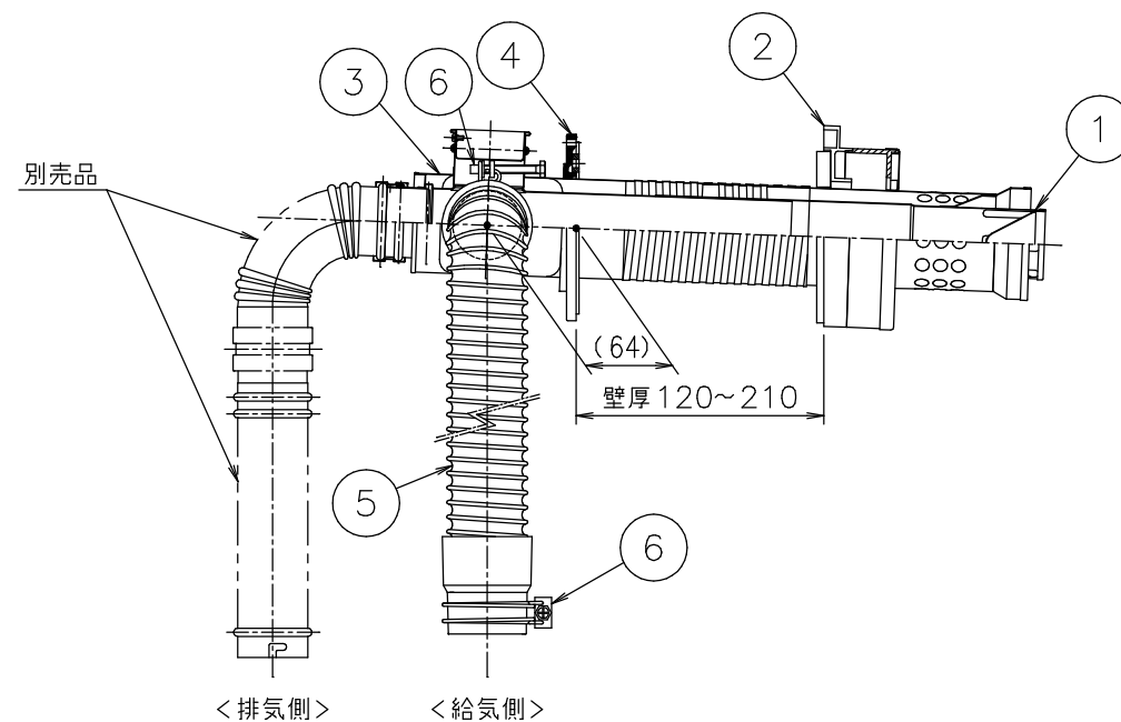
側面図
