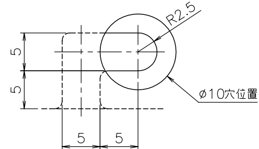
■ A部詳細図 (尺度 2/1)
