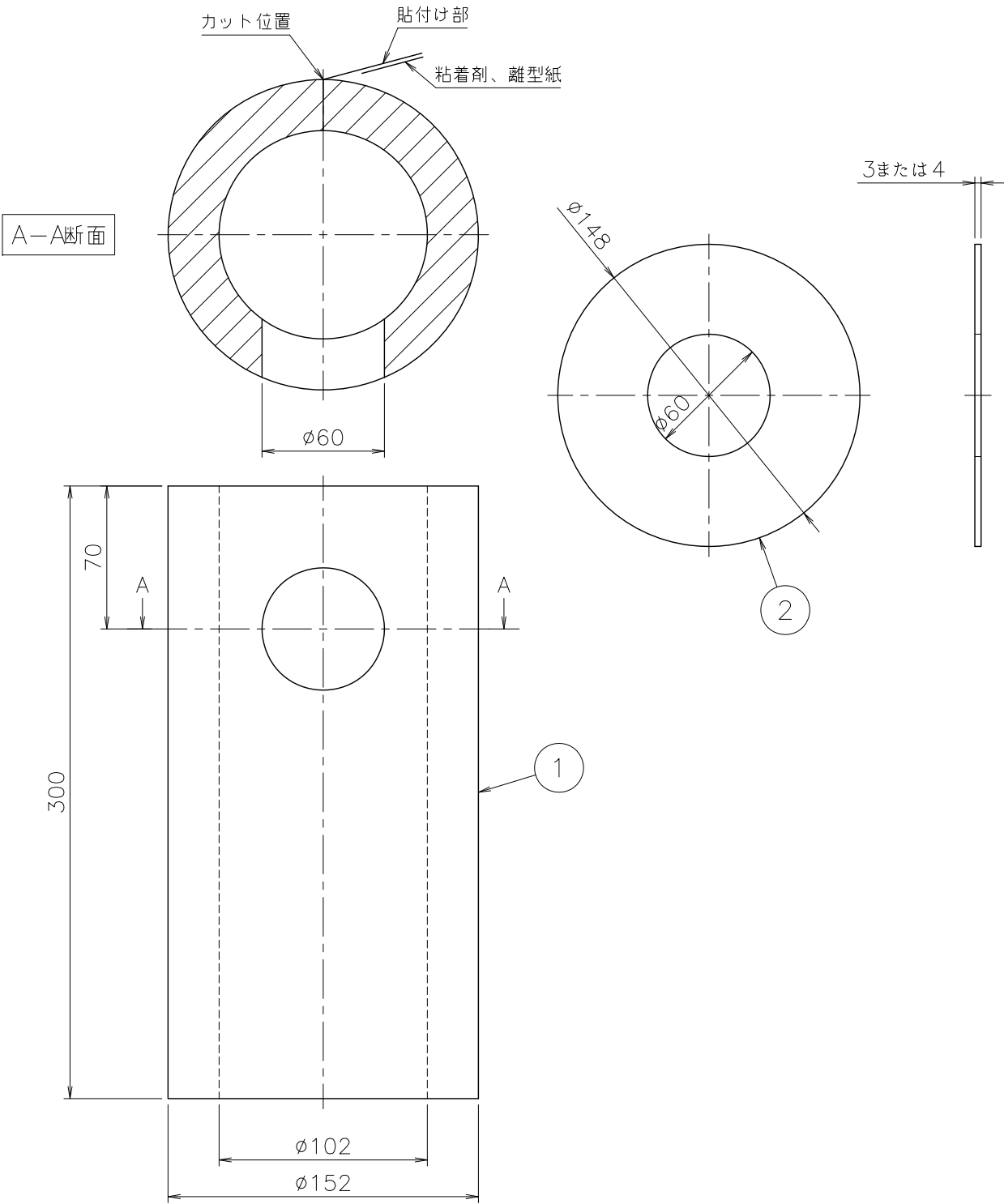
■φ49給排気筒保温材セット VK-HZ-02E
