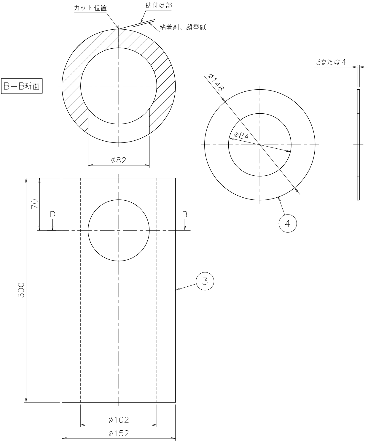
■φ70給排気筒保温材セット VK-HZ-091
