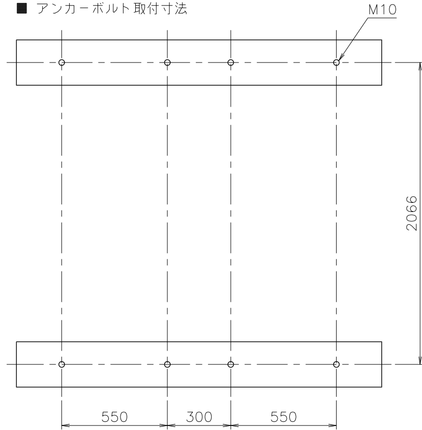
■ アンカーボルト取付寸法
