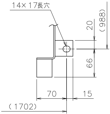
アンカー固定部詳細 (A部)
