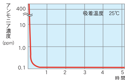
フレッシュドライのアンモニア吸着力
