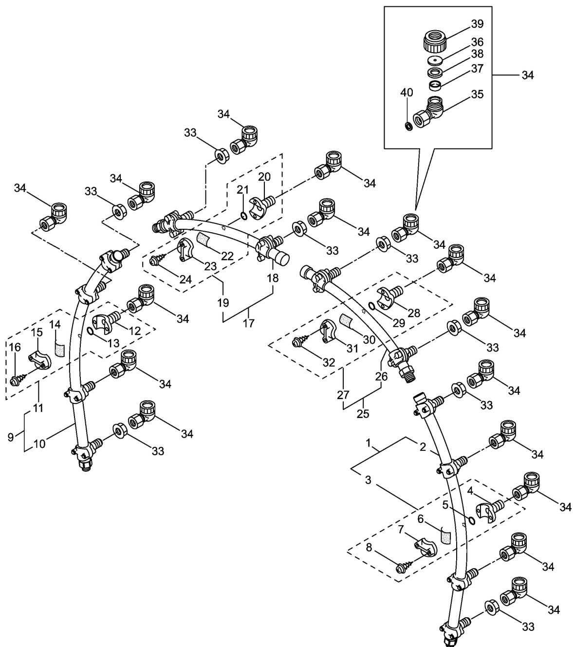
ノズル配列図
