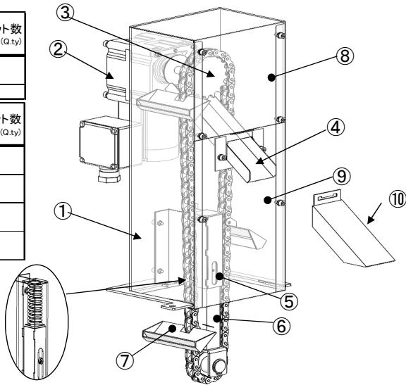
内部詳細図
