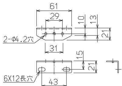
取付金具下(左右共通) (尺度フリー)
