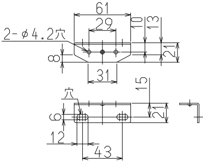
取付金具下 (左右共通) 尺度:フリー
