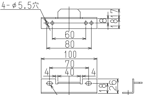
取付金具上 尺度:フリー
