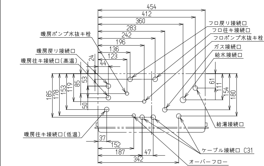
〔上方からの透視図〕
