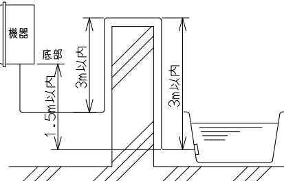
●トリイ配管を行う場合
