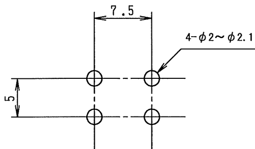
基板加工例
