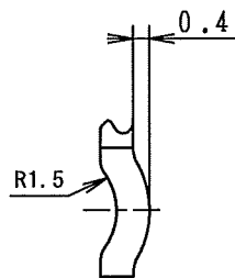
A部詳細図 (S=5/1)
