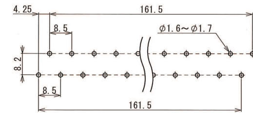
プリント基板穴寸法
